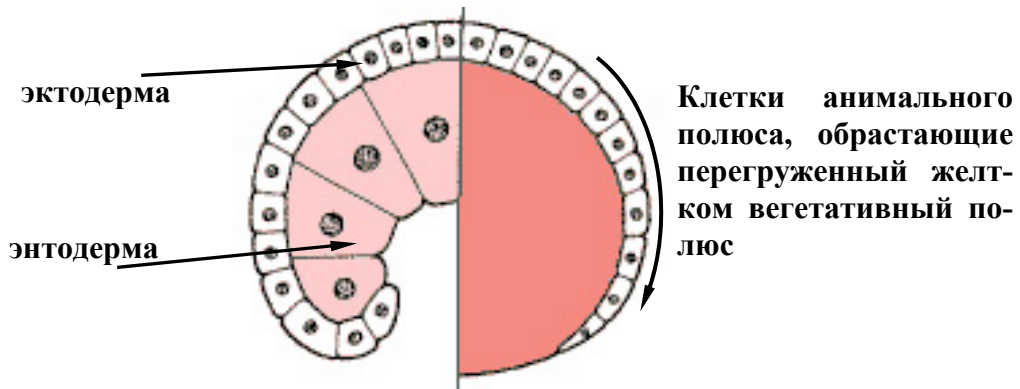
Рис. 5. Эпиболия (схема)
