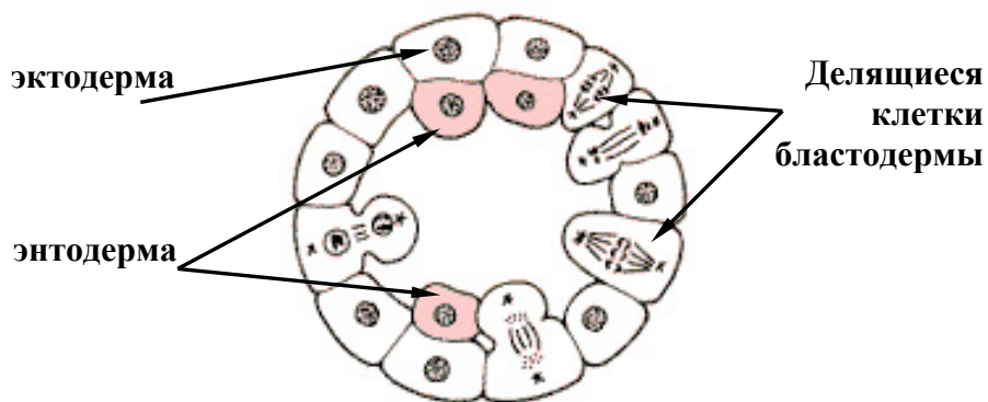
Рис. 4. Деляминация (схема)
