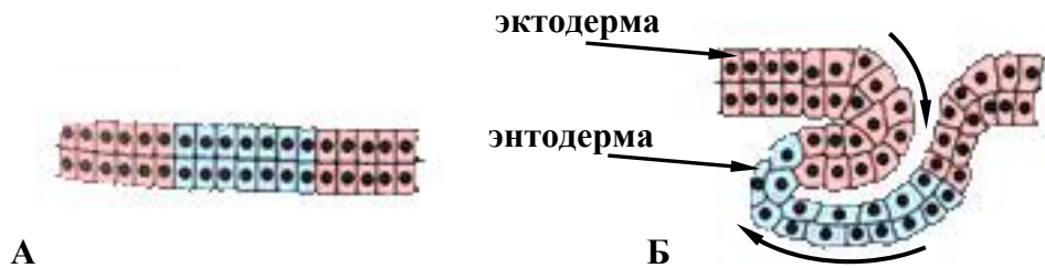
Рис. 2. Схема инволюции:
