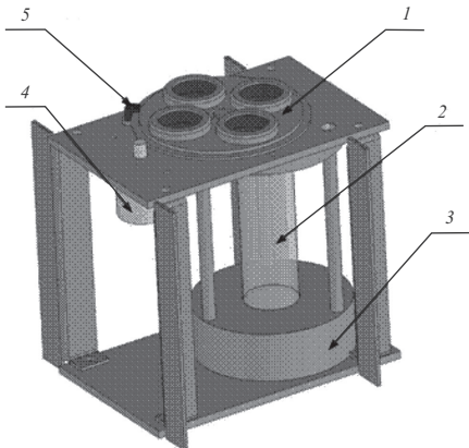
Рис. 17. Эскиз системы спектральной селекции надводного модуля: 1 – револьверная головка с набором светофильтров; 2 – ФЭУ-142; 3 – делитель ФЭУ; 4 – шаговый двигатель; 5 – оптопара
