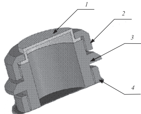
Рис. 18. Конструкция входного коллектора излучения: 1 – входной коллектор; 2 – верхнее прижимное кольцо; 3 – основание; 4 – нижнее прижимное кольцо
