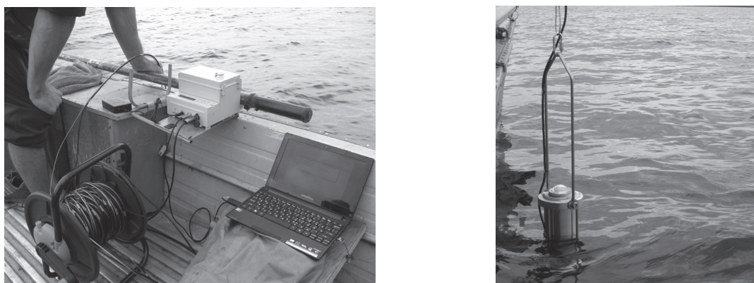
Рис. 27. Испытания погружного прибора на оз. Нарочь
