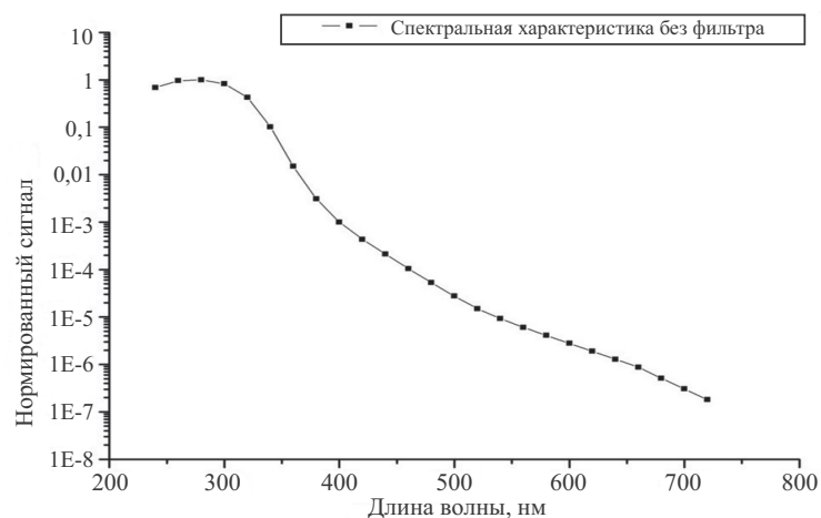
Рис. 25. Спектральная характеристика надводной части прибора без фильтра
