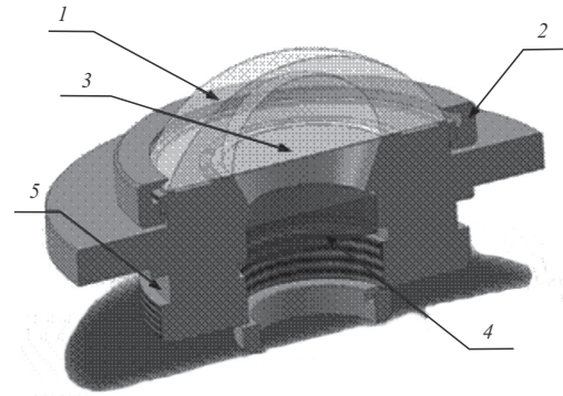
Рис. 15. Входной коллектор излучения с широкоугольным объективом типа «рыбий глаз»: 1 – кварцевая линза; 2 – прижимное кольцо; 3 – тефлоновый рассеиватель; 4 – светофильтр; 5 – паз для уплотнительного кольца
