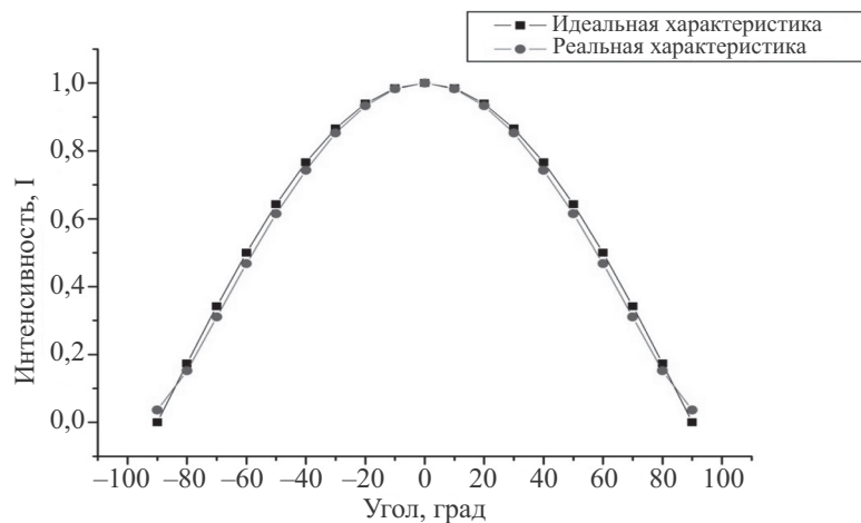
Рис. 22. Угловая характеристика надводной части прибора
