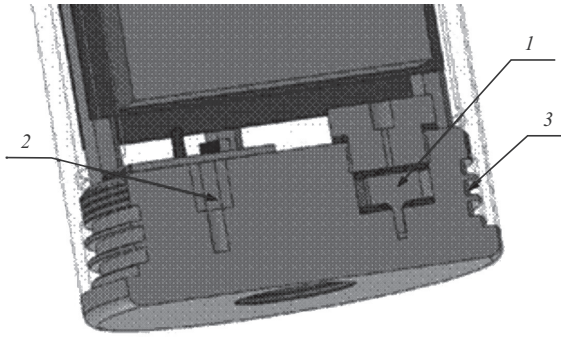
Рис. 14. Конструкция крышки основания: 1 – датчик давления воды; 2 – датчик температуры воды; 3 – пазы для уплотнительных колец
